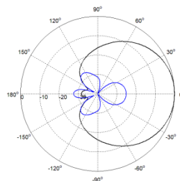
垂直方向图
