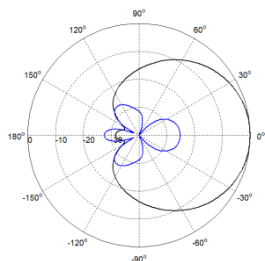
水平方向图
