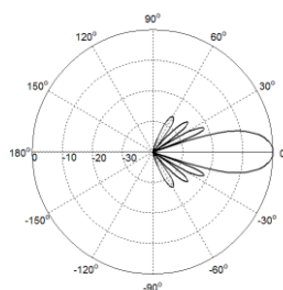
垂直方向图
