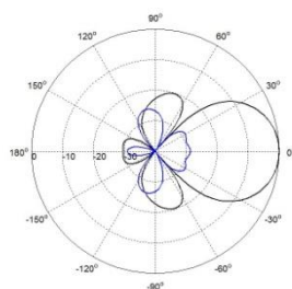
垂直方向图
